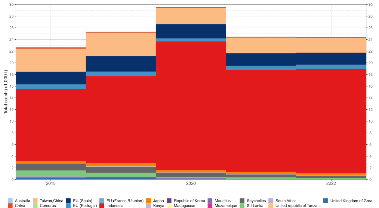
Figure 2 : Séries temporelles annuelles des captures retenues (en tonnes ; t) de requin peau bleue par flottille pour la période 2018-2022. Il existe de grandes incertitudes liées aux estimations des captures de requin peau bleue des pêcheries artisanales indonésiennes. La révision de la composition des captures des pêcheries indonésiennes est en cours.
