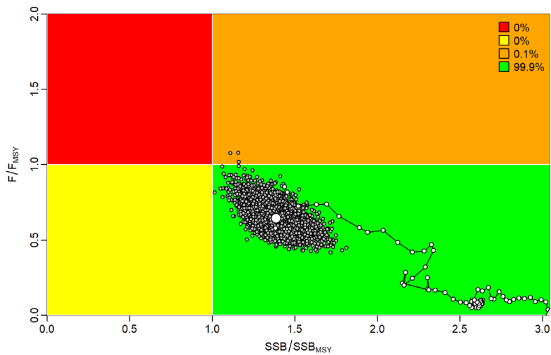
Fig. A 1. Requin peau bleue : Diagramme de Kobe de l'évaluation du stock agrégée pour l'océan Indien d'après le cas de base du modèle de l'évaluation de 2021 (cas de base du modèle comportant la trajectoire et les incertitudes pour l'année finale).
