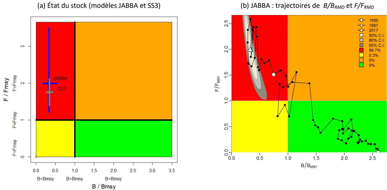
Figure 2. Marlin rayé : (a) État du stock selon l'évaluation pour l'océan Indien, modèles JABBA (modèle bayésien d'espace d'état de production excédentaire) et SS3 avec intervalles de confiance (à gauche) ; (b) Trajectoires (1950-2017) de B/B_{RMD} et F/F_{RMD} d'après le modèle JABBA. NB : SS3 se réfère à SB/SB_{RMD} alors que la sortie du modèle JABBA se réfère à B/B_{RMD} .
