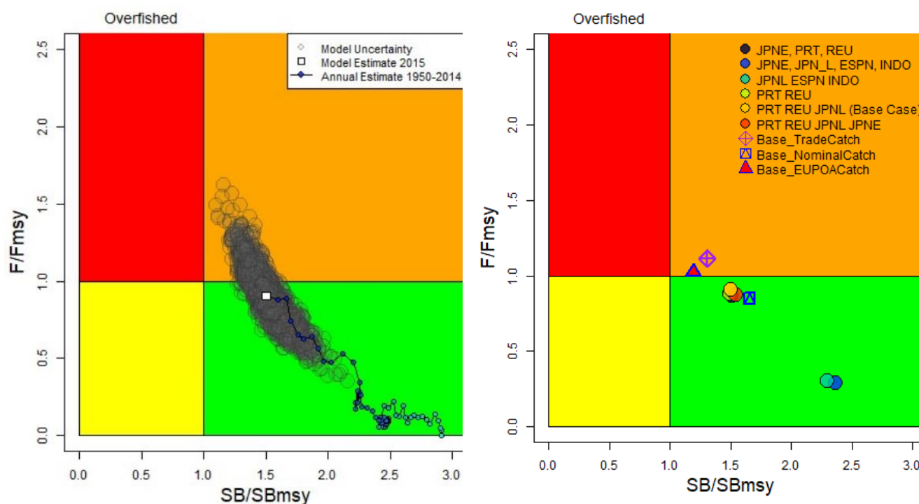
Figure 1. Requin peau bleue : Diagramme de Kobe de l'évaluation de stock appliquée à l'ensemble de l'océan Indien, réalisée avec les estimations 2017 issues du modèle de référence et de plusieurs modèles de sensibilité explorés avec plusieurs reconstructions des prises et des ajustements des séries de PUE. (À gauche : modèle de référence comportant la trajectoire et les incertitudes MCMC pour l'année finale ; à droite : estimations des scénarios de sensibilité des modèles pour l'année finale). Tous les modèles présentés utilisent SS3 - Stock Synthesis III.
