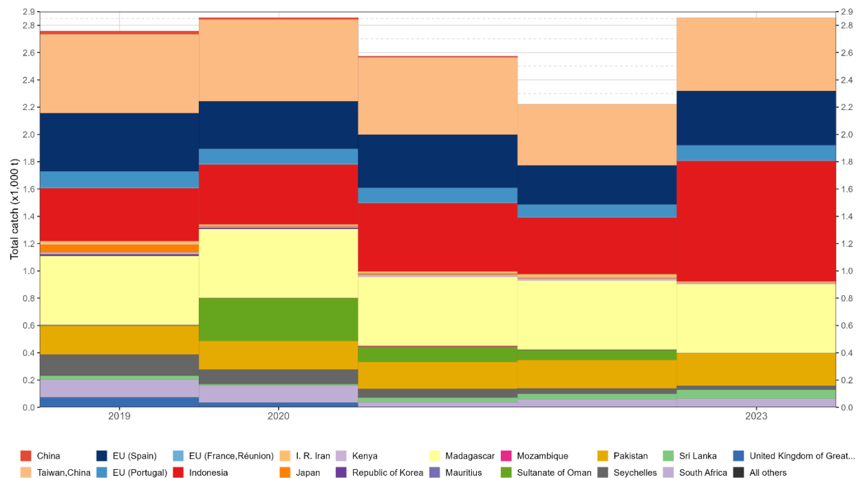
Fig 2. Séries temporelles annuelles des captures retenues (tonnes ; t) de requin-taupo bleu déclarées au niveau de l'espèce ou agrégées (SMA, MAK et MSK) par flottille pour la période 1919-2023.
