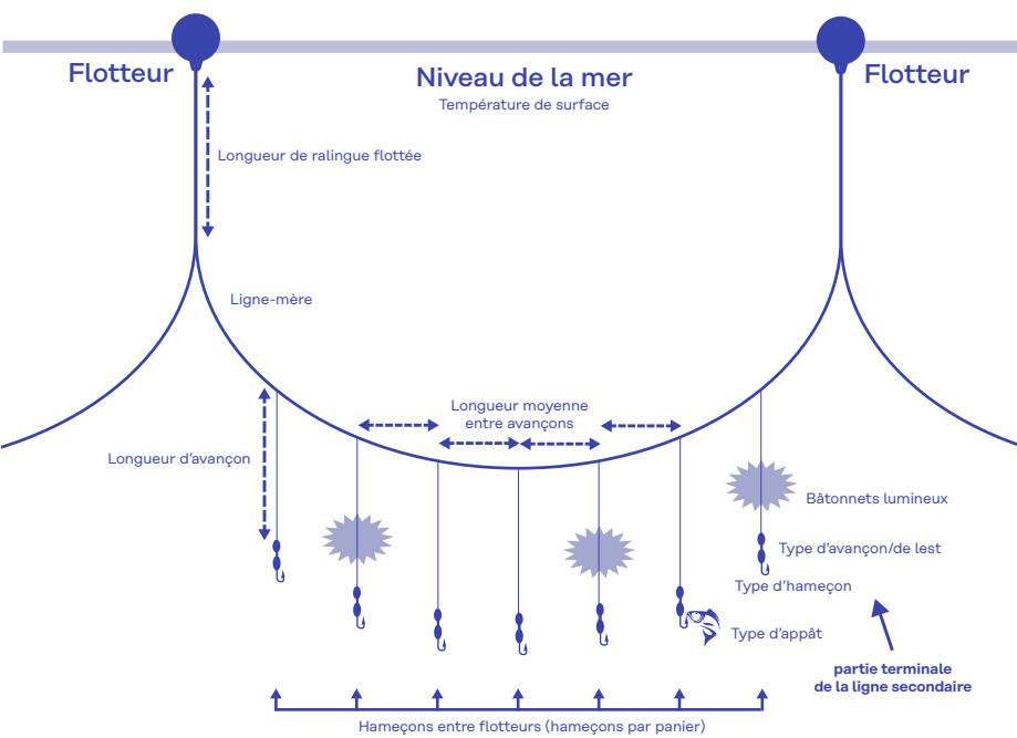
Figure 1. Représentation schématique d'une palangre. Longueur moyenne des avançons (mètres): longueur droite entre l'agrafe et l'hameçon.
