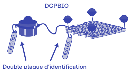
Schéma de la procédure de fixation du numéro d'identification du DCPbio affiché sur la plaque métallique au radeau et à la bouée échosondeur associée.
