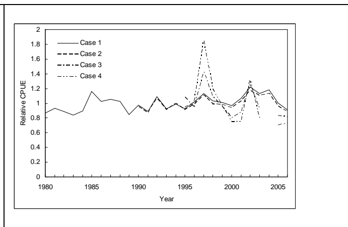
Figure 6 : Tendances de la PUE normalisée pour les espadons capturés par les palangriers taiwanais dans l'ensemble de l'océan Indien, dérivées selon quatre scénarios. La PUE nominale est également indiquée.
