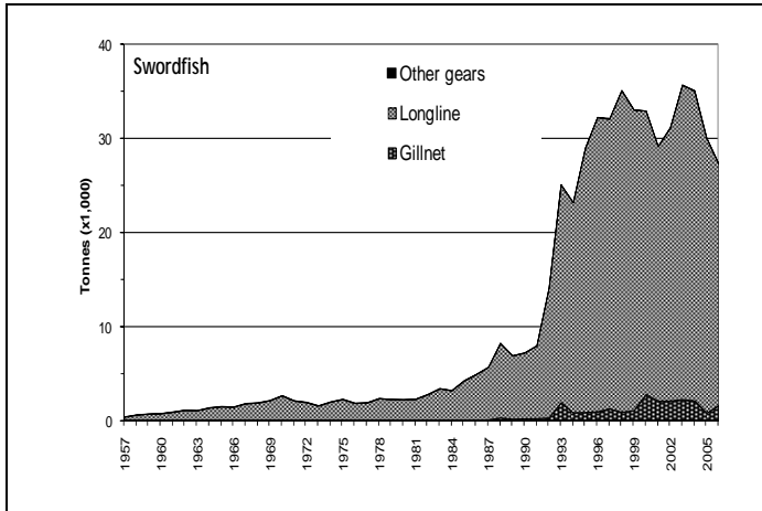
Figure 3. Captures d'espadon par engin et par an enregistrées dans les bases de données de la CTOI (1957-2006). Données en date de juillet 2008
