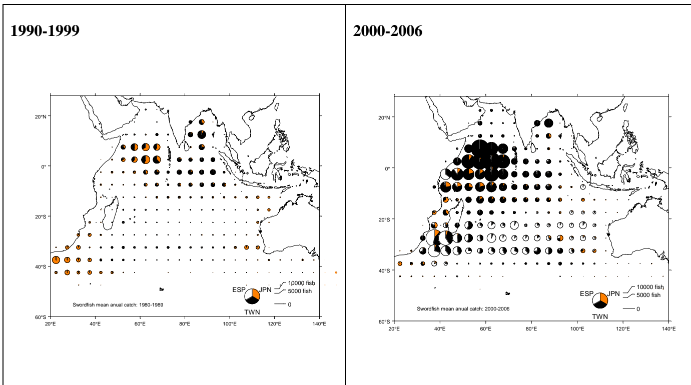
Figure 4. prises annuelles moyennes d'espadon (tonnes) entre 1990 et 1999 et entre 2000 et 2006 pour les palangres, les filets maillants et les autres pêcheries dans l'océan Indien.
