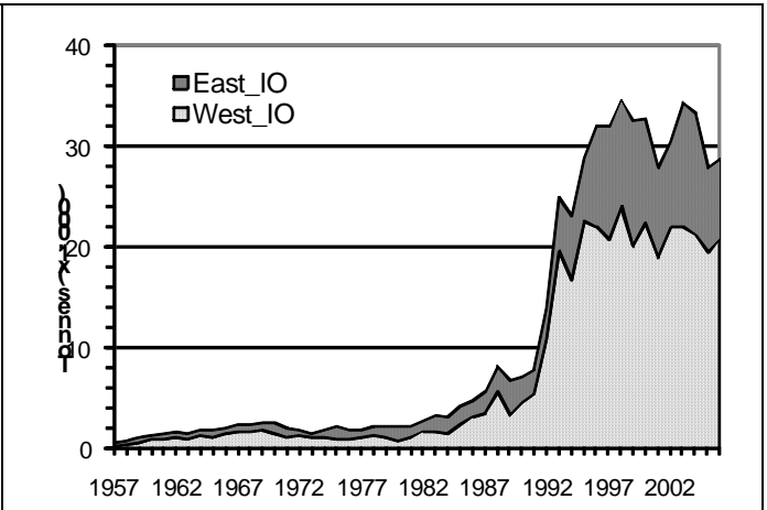
Figure 4. Évolution des prises d'espadon dans les zones ouest et est de l'océan Indien entre 1957 et 2006. Données en date de juillet 2008
