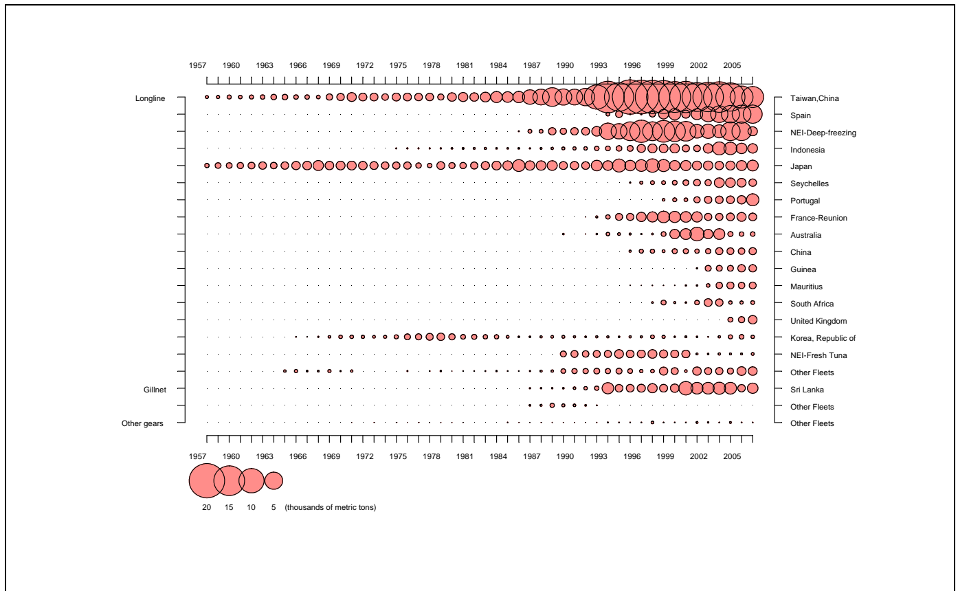
Figure 3. Captures d'espadon par engin et pays/flotte dans l'océan Indien entre 1957 et 2006, en millier de tonnes. Données en date d'juillet 2008
